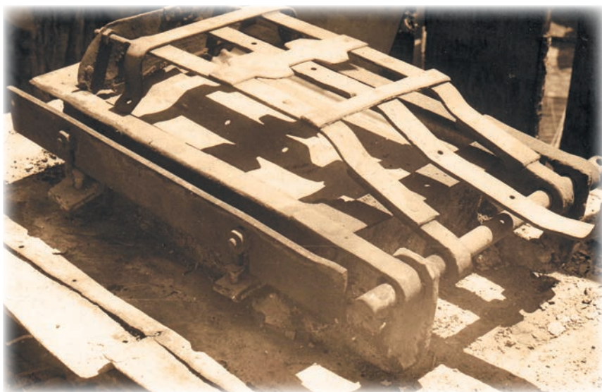
Станок для отформовки плоской глиняной черепицы (архив М.В. Маруневич)
