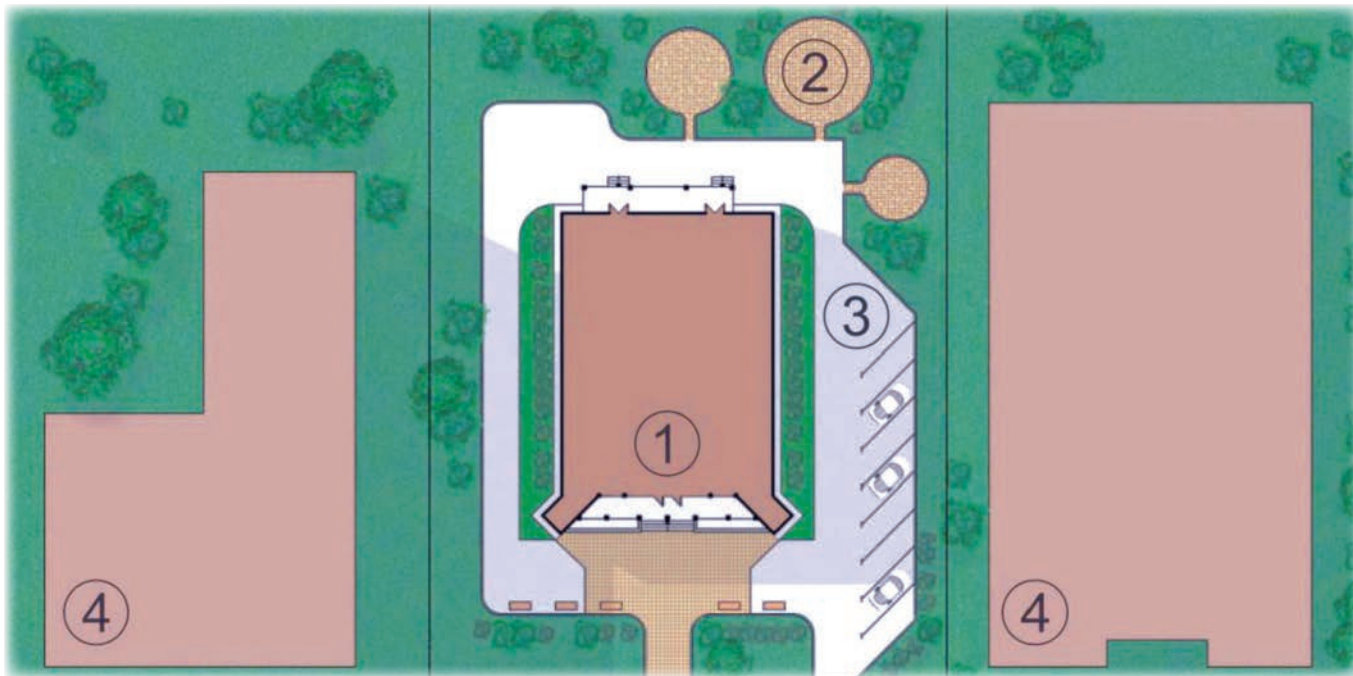
Схема генерального плана. 1 - проектируемое здание; 2 - площадки для отдыха; 3 - временная парковка; 4 - существующие здания. Площадь участка - 0,41 га.
