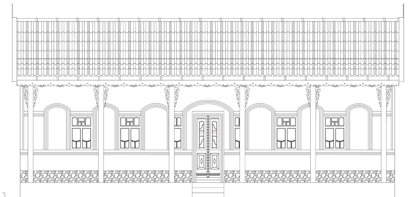
Графическая модель традиционного гагаузского жилища Adetçä gagauz yaşamak erin grafika modeli
