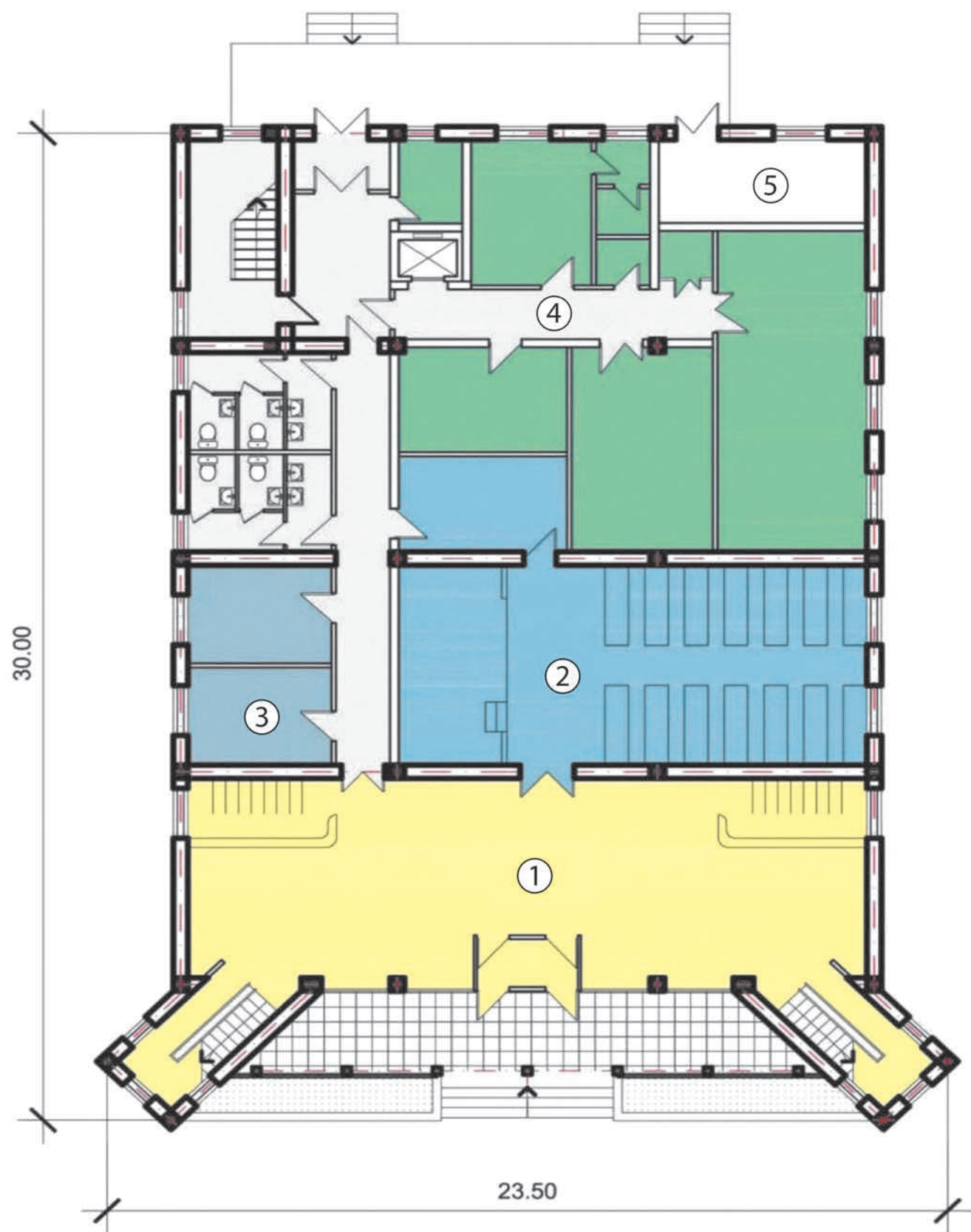
План первого этажа: 1 - вестибюль-фойе; 2 - конференц-зал; 3 - администрация; 4 - помещения кухни; 5 - котельная
